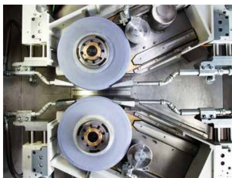
Zwei-Spindel Variante
