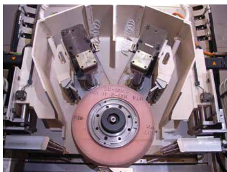
Überkopf-Einrollgerät
