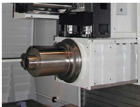
Überkopfabrichtgerät bis 300 mm Breite
