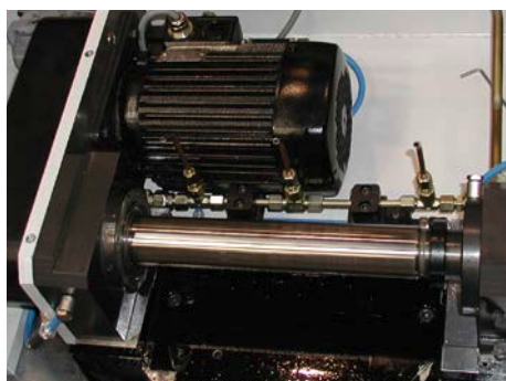
Tischmontiertes Profileinrollgerät
